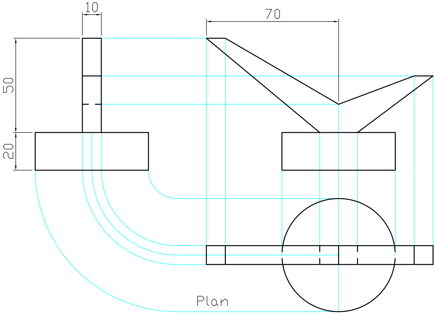
End Elevation
