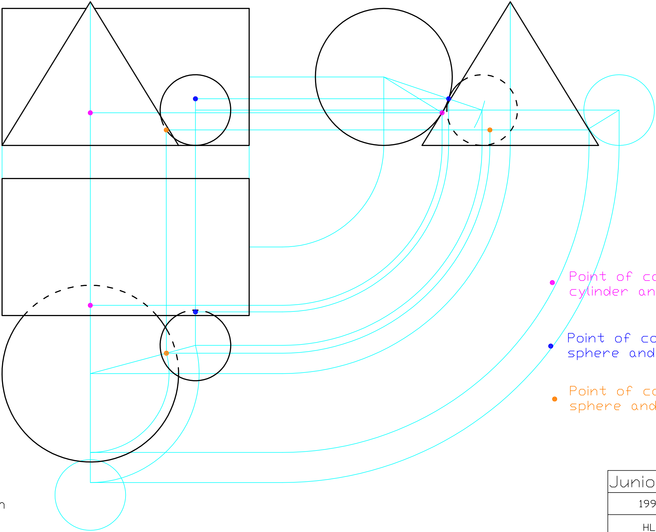
End Elevation
